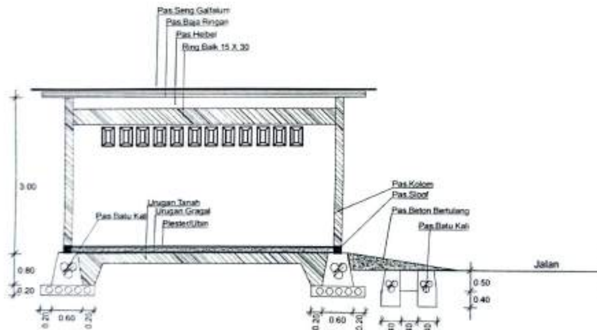
POT B - B SKALA 1 : 50
